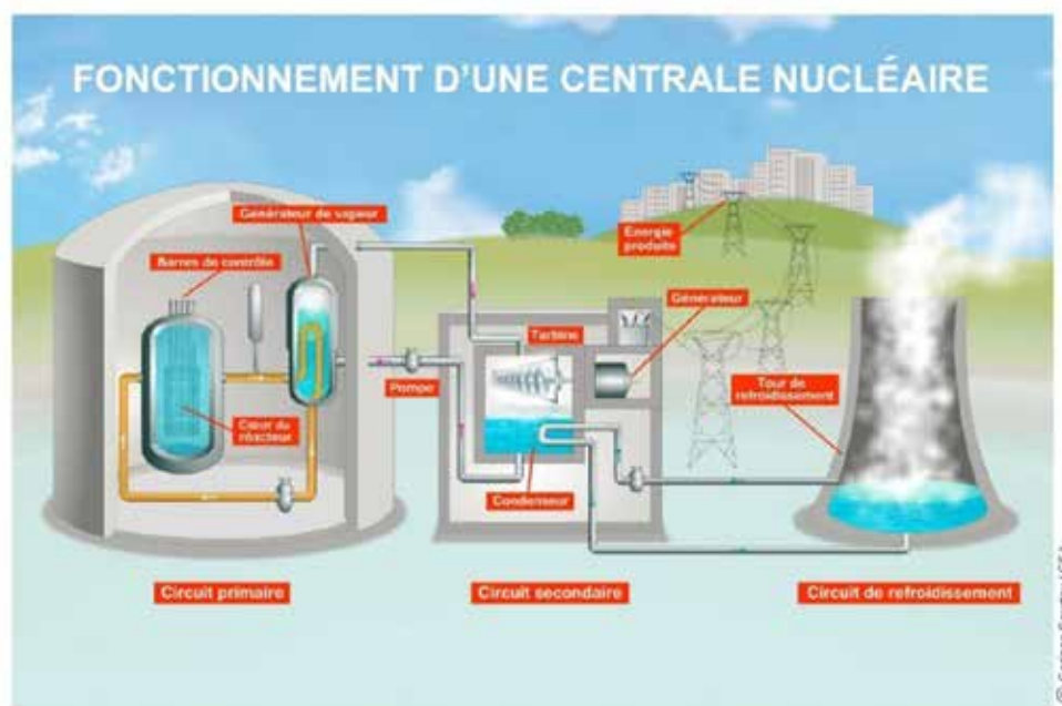
Figure : Fonctionnement d'une centrale nucléaire ; source : CEA
