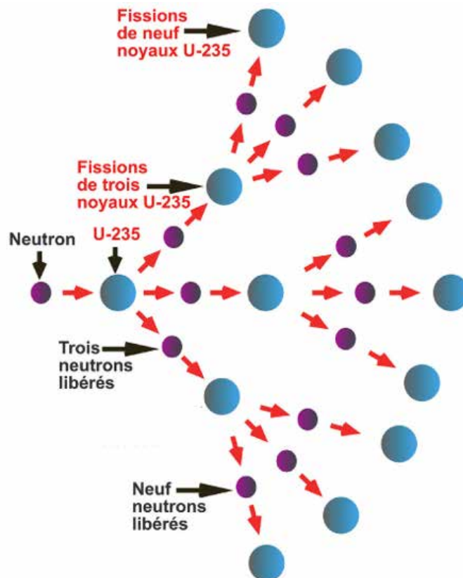
Figure : Réaction en chaîne au sein des réacteurs ; source : ResearchGate
